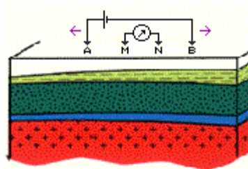
Variation de la résistivité avec la profondeur
