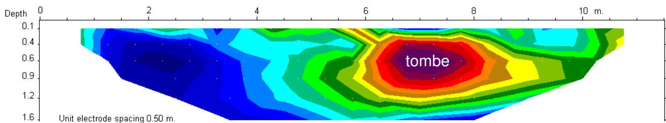
Anomalie résistante au dessus d'une ancienne tombe sur un site romain (inversion 2D en Wenner)
